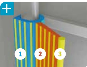
JOINTS PÉRIPHÉRIQUES TRIMATIERE* Développé par France Fermetures pour équiper ses portes sectionnelles plafond, ce joint assure l'étanchéité périphérique de la porte. Il se compose de 3 matières qui garantissent : la tenue du joint (1 Embase rigide), l'étanchéité de la porte (2 Lèvre souple) et la souplesse de fonctionnement (3 Agents glissants).
