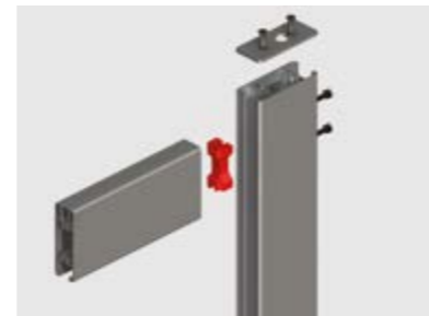
Assemblage mécanique
